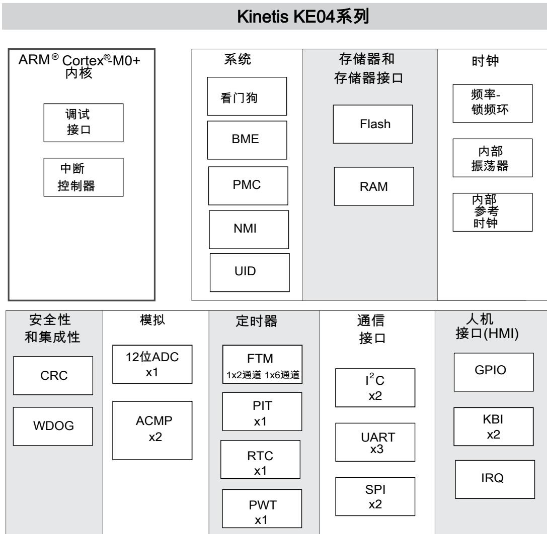
图 1. KE04 系列功能框图
