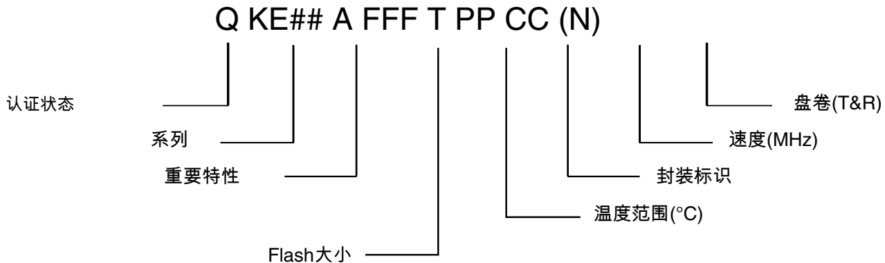
图 2. 部件编号图
