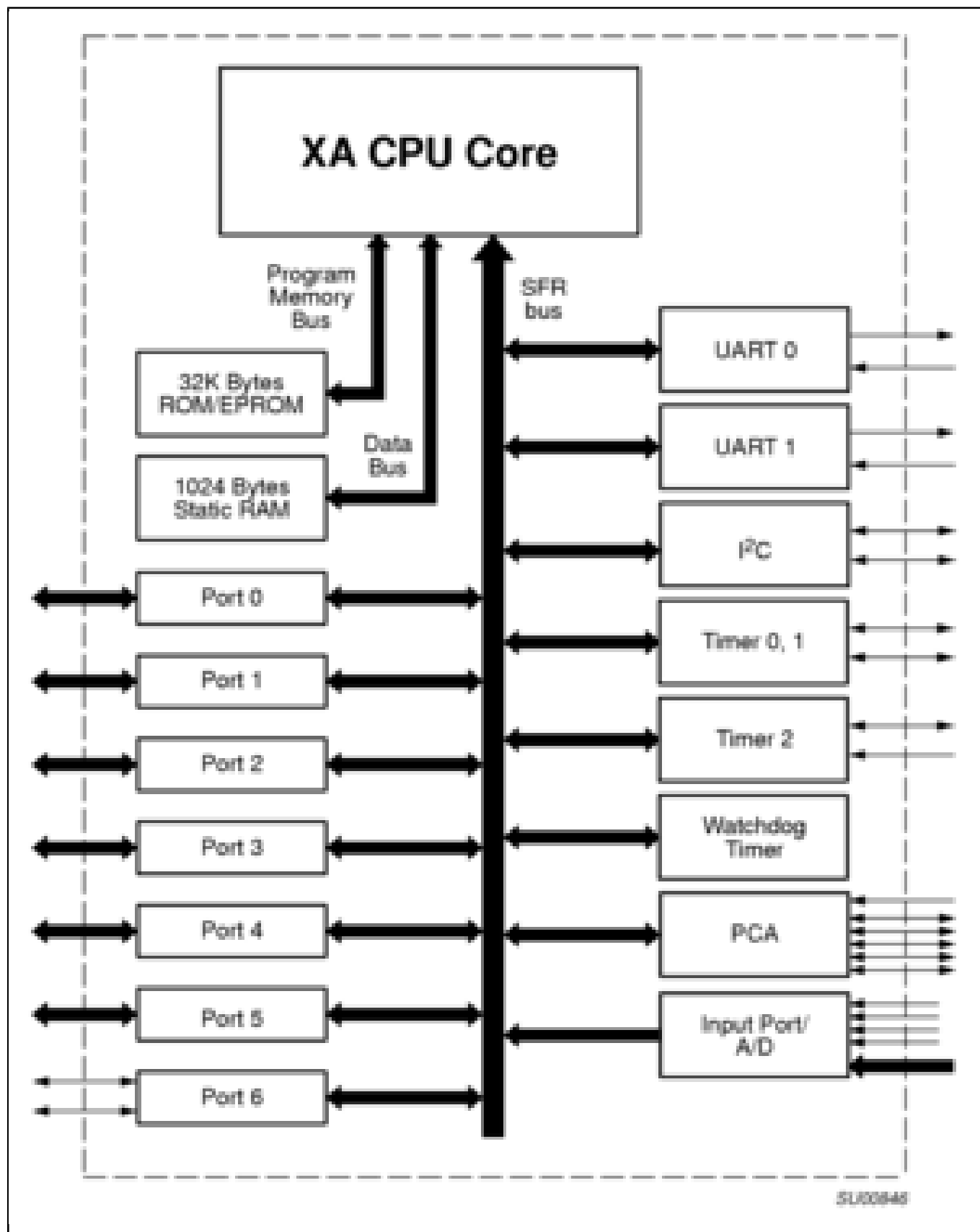
Block diagram: PXAS30KBA, PXAS30KBBE, PXAS30KFA, PXAS37KBA, PXAS37KBBE Block Diagram
