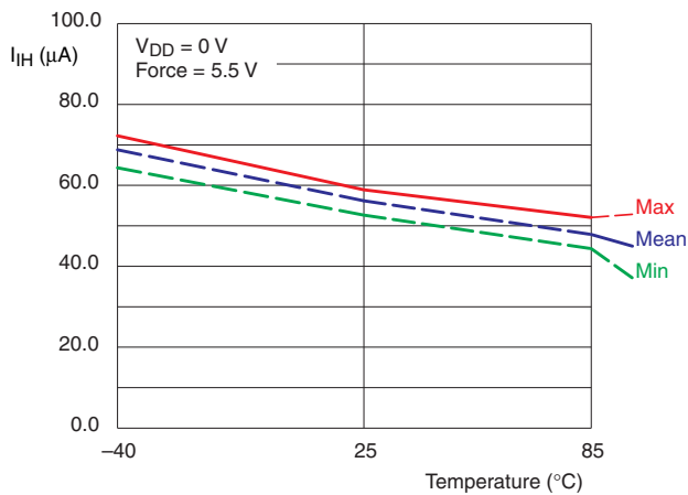
Fig 27. PCA9535 I/O leakage when V DD = 0 V
