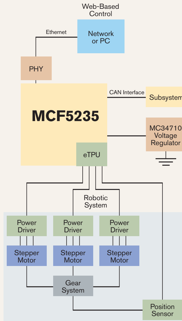
MCF523x BLOCK DIAGRAM
