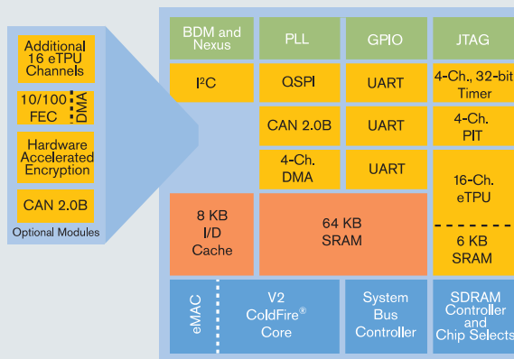
MCF523x BLOCK DIAGRAM
