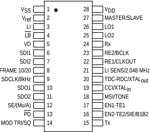
28-PIN SOIC/TSSOP PACKAGES
