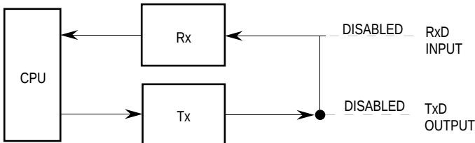
(b) Local Loopback
