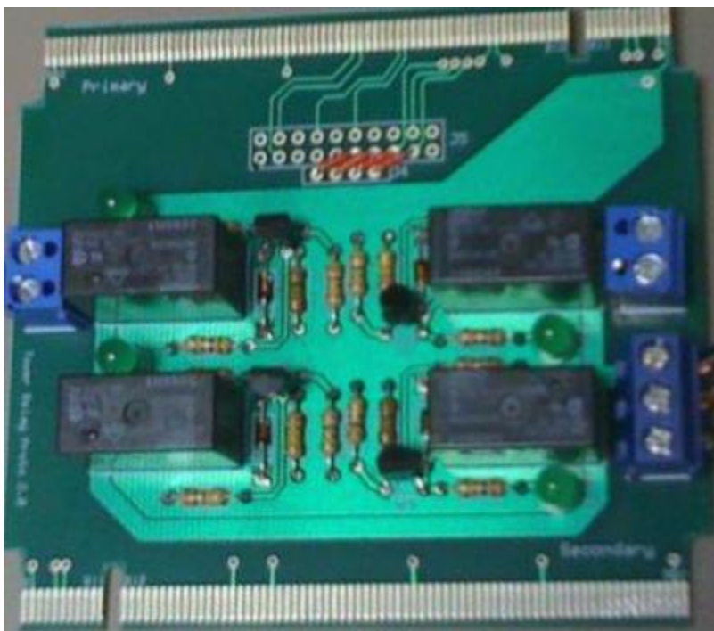
图 3. 继电器模块
