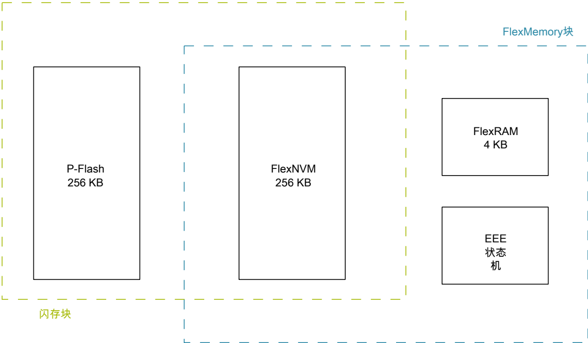
图 8. Kinetis flash 块
