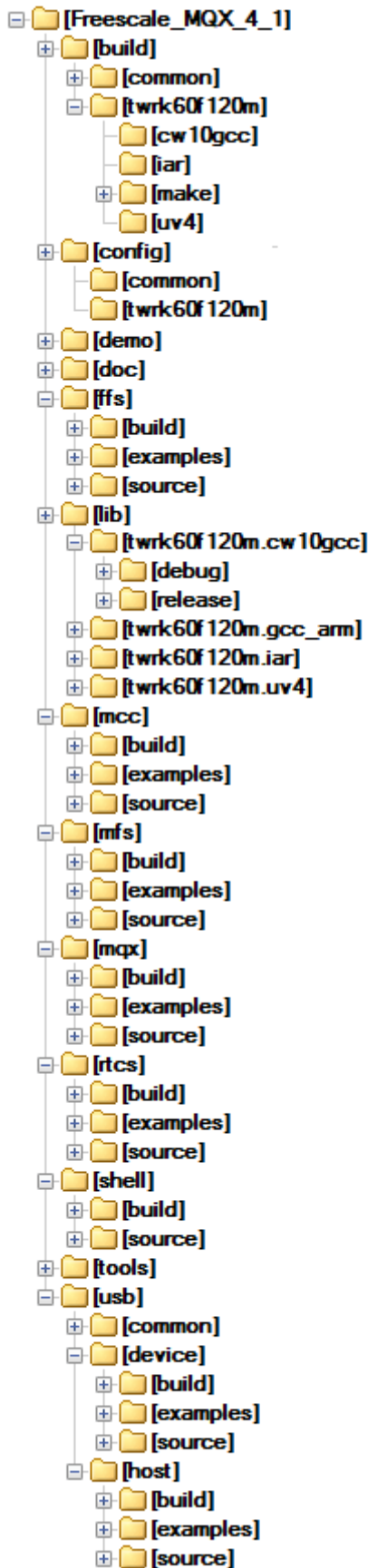
图 4-1. Freescale MQX RTOS 目录结构 Freescale MQX™ RTOS for Kinetis SDK 用户指南, Rev. 2, 04/2015
