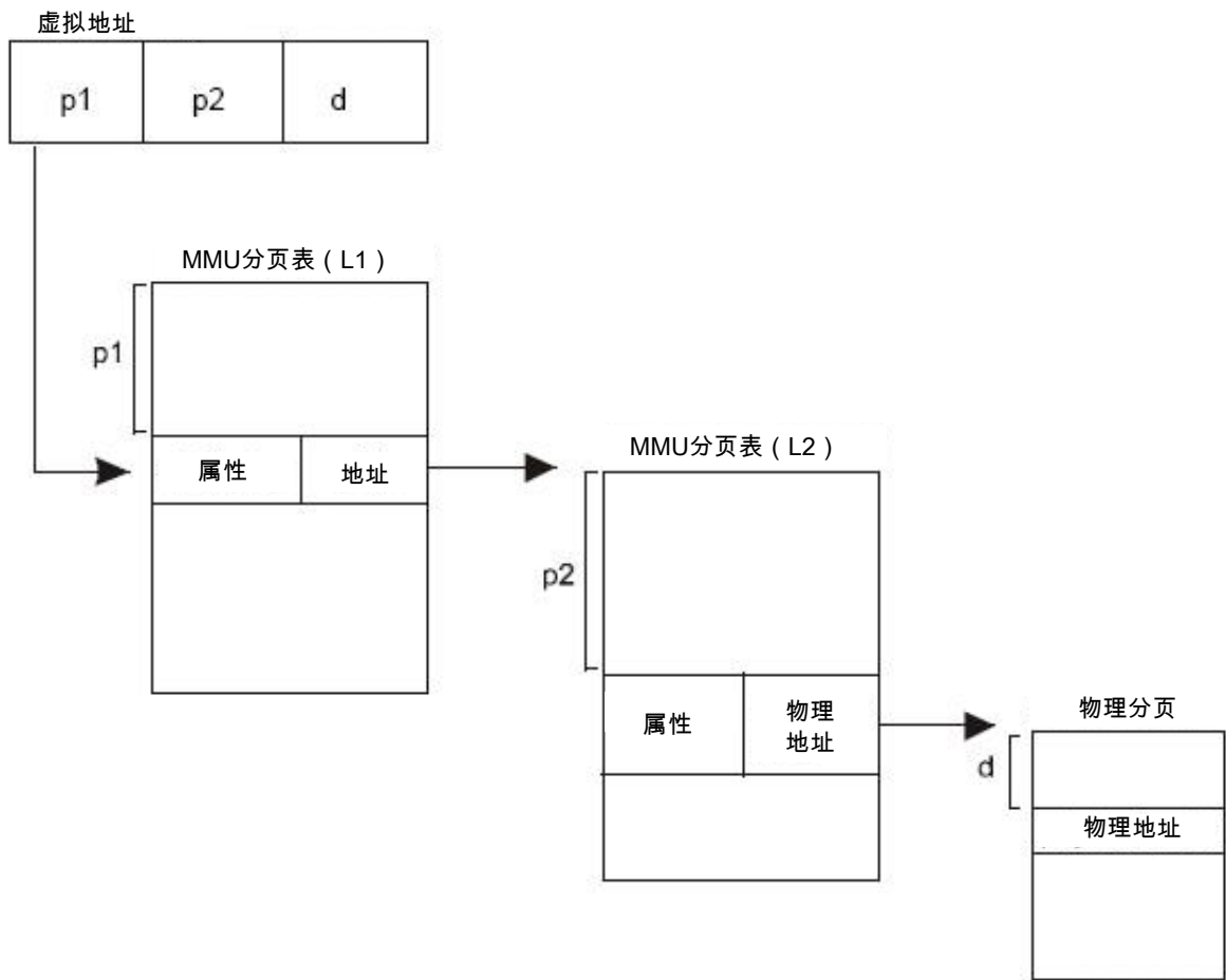
图 3-2. 虚拟和物理地址。
