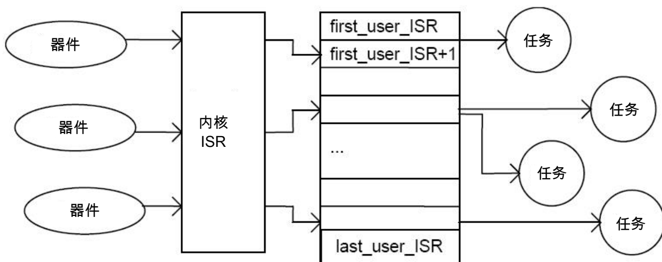
图 3-3. 处理中断
